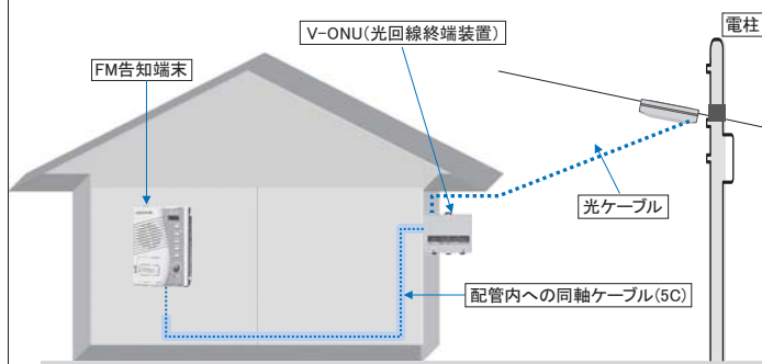
機器設置写真(参考)
