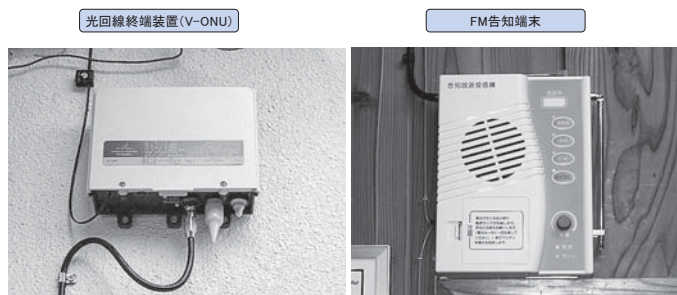
機器設置写真(参考)
