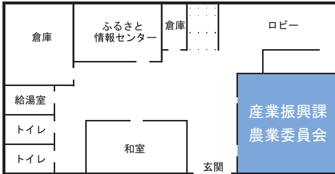
農村環境改善センター 1階平面図
