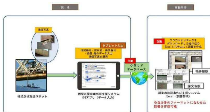
図 5.1.1 点検後の調書・図面作成に対する新技術（例：点検調書、図面支援システム）
